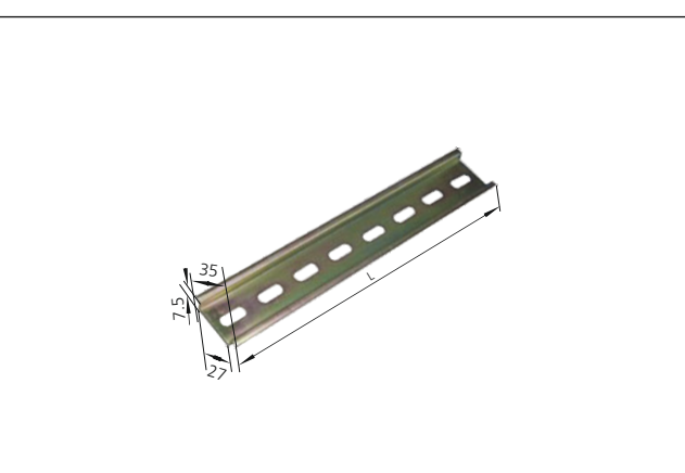
Fig. 3 Guida DIN di installazione
